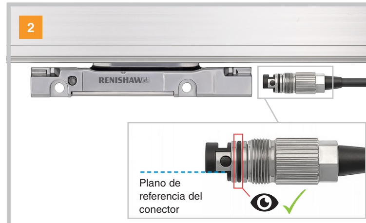
Introduzca el cable en la cabeza lectora. Compruebe la orientación correcta del conector: el plano de referencia debe estar orientado hacia la base de la cabeza lectora.
