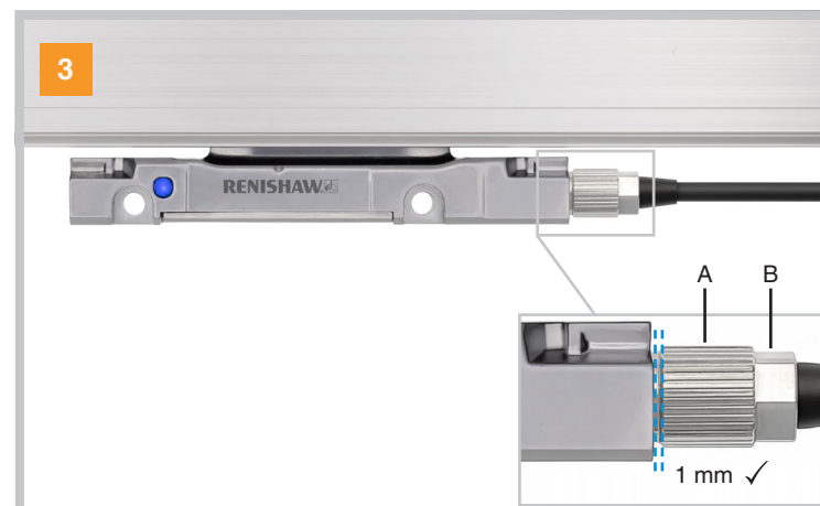
Enchufe el conector en la toma y apriete a mano la rosca "A".
